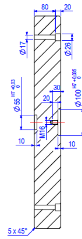
KESİT H-H
